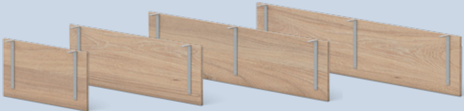
VENO-903-1 | 903-2 | 903-3 | 903-4 18×700×350 | 1100×350 | 1500×350 | 1700×350 mm
