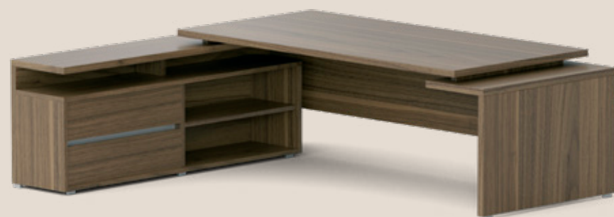
EXO-710-3 2400×2000×750 mm
